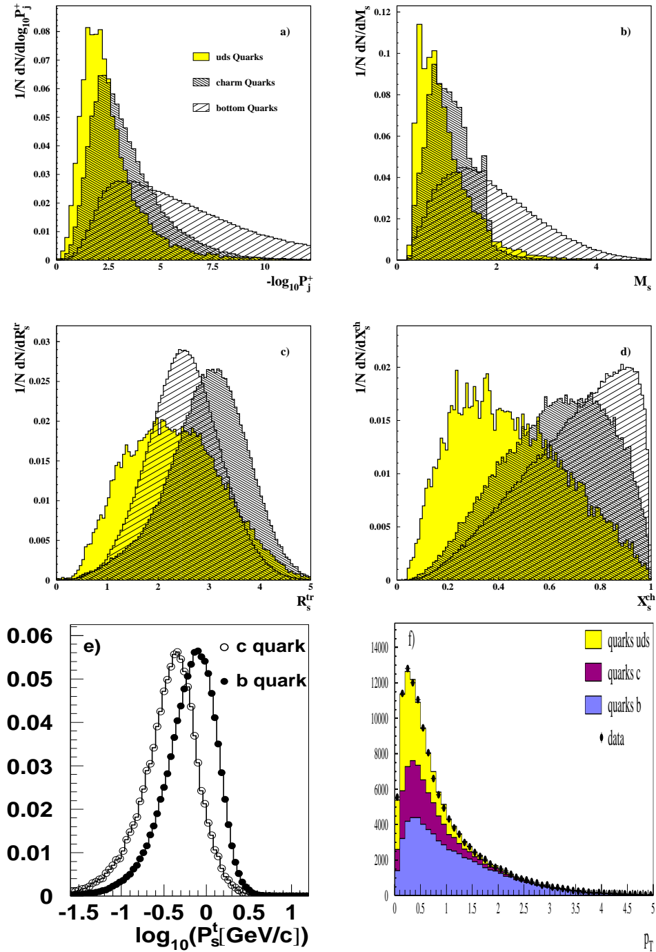
Abbildung 4.2: Die Diskriminanzvariablen zur Berechnung des b_{\text{tag}} . a) Wahrscheinlichkeit P_j^+ aus der Lebensdauerinformation, b) effektive Masse M_s , c) Rapidität R_s^{\text{tr}} , d) Energieanteil X_s^{\text{ch}} [47]. e) Logarithmus aus den Transversalimpuls der Spuren des sekundären Vertex \log_{10}(P_s^t) [49]. f) Transversalimpuls P_T von identifizierten Leptonen [48, 49].
