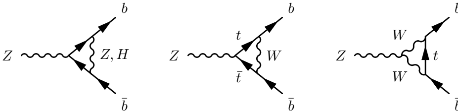
Abbildung 2.7: Die Vertexkorrekturen.
