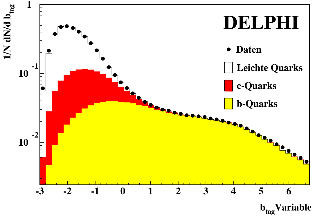
Abbildung 4.4: Die b_{\text{tag}} -Verteilung der verbesserten Impaktparameter-Methode für das Jahr 1994.
