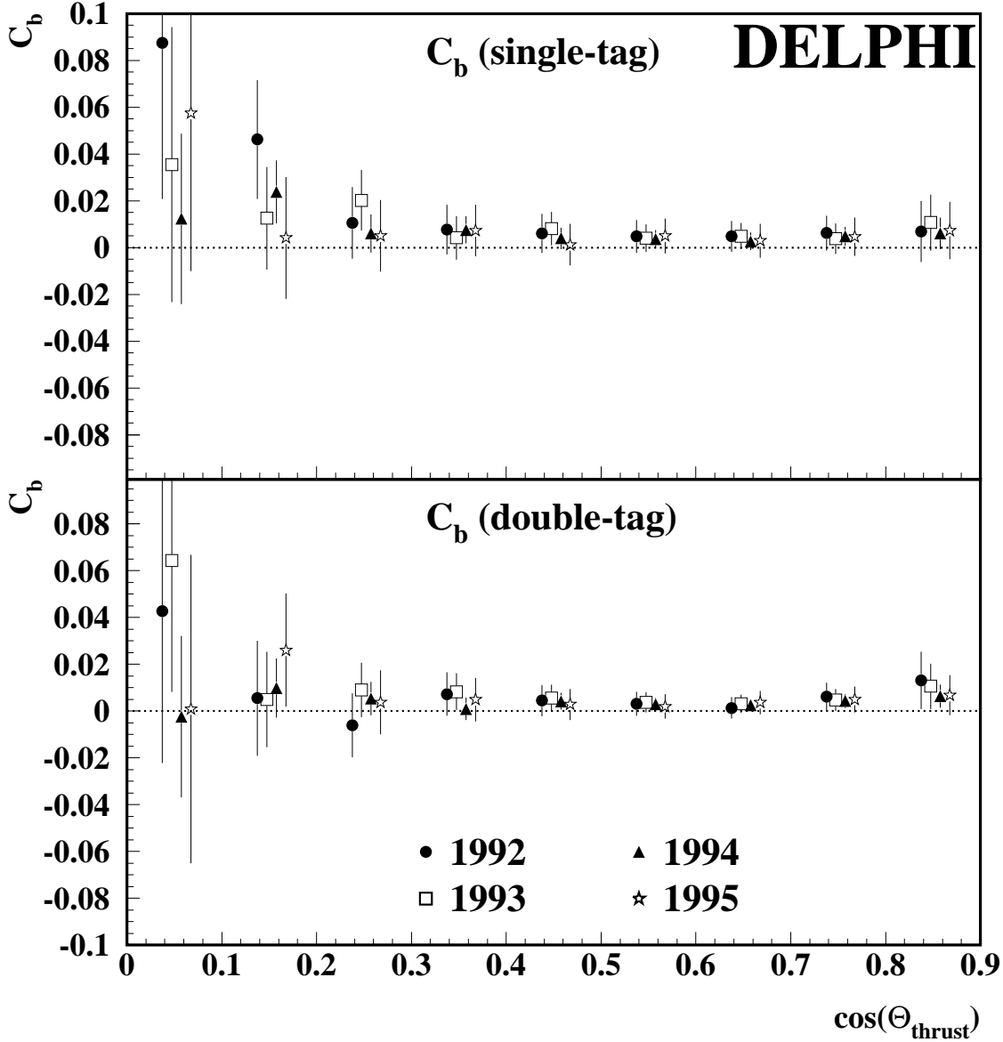
Abbildung 5.2: Der Koeffizient der QCD-Korrektur C_b = s_b C_{QCD}^{b,jetset} , der den experimentellen Bias s_b der QCD-Korrektur C_{QCD}^{b,jetset} berücksichtigt als Funktion des Polarwinkels der Thrustachse. In der oberen Abbildung ist die Korrektur der single-tagged Ereignisse, in der unteren Abbildung die der double-tagged Ereignisse zu sehen. Angewendete Selektionsschnitte: b_{\text{tag},1992-1993} > -0.1 , b_{\text{tag},1994-1995} > 0.1 , |flav_{\text{hem}}| > 0.35 .
