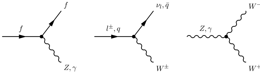
Abbildung 2.1: Die fundamentalen Feynmandiagramme der elektroschwachen Theorie.
