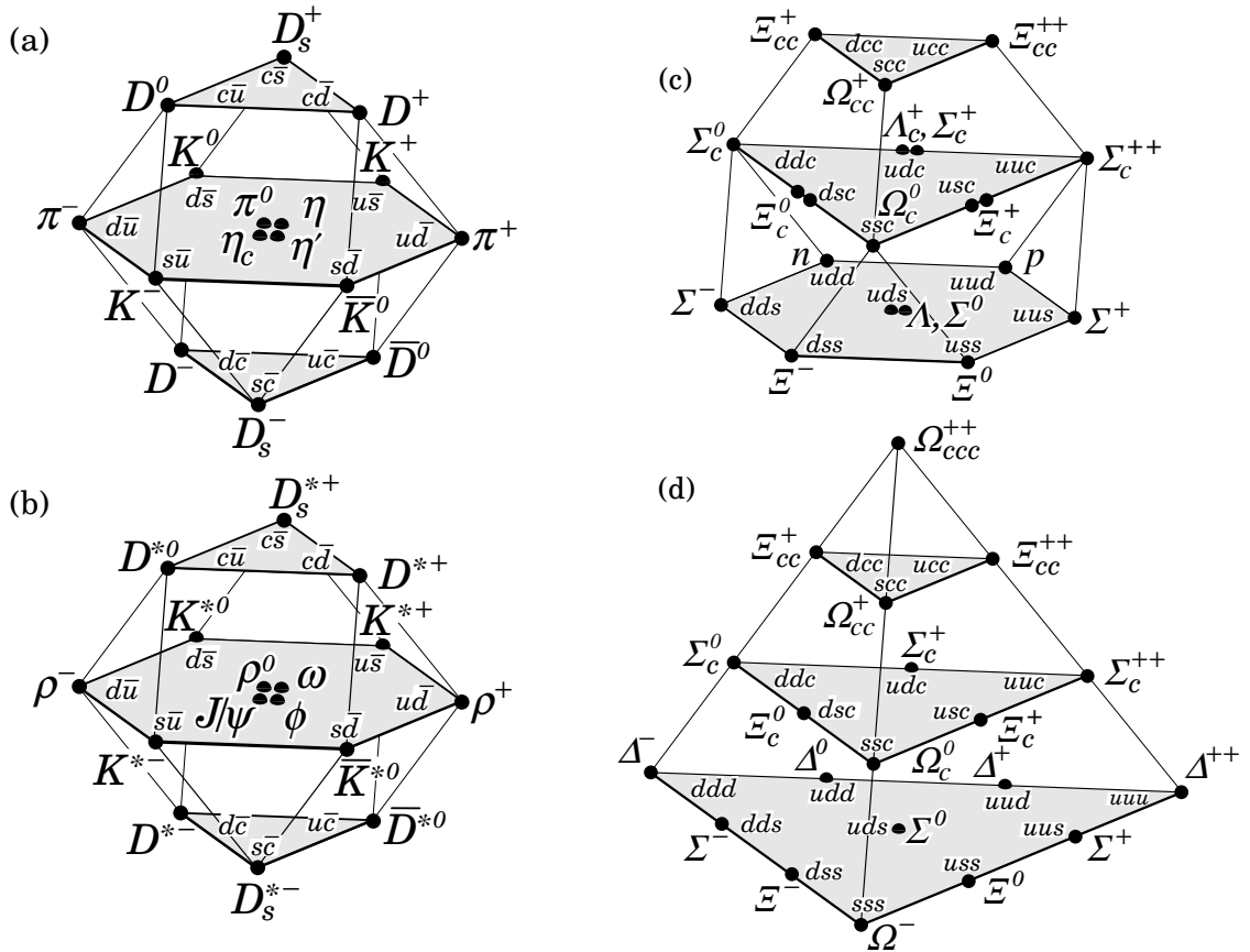
Abbildung 2.11: Die Zusammensetzung der Meson- und Baryonmultiplikts aus d -, u -, s - und c -Quarks für pseudoskalare (a) und Vektormesonen (b) bzw. für Baryonen mit Spin \frac{1}{2} (c) und Spin \frac{3}{2} (d) [32].
