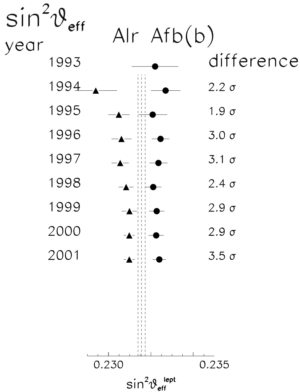
Abbildung 6.3: Zeitliche Entwicklung der Asymmetriemessungen. Die Sommerkonferenzwerte der Links-Rechts-Asymmetrie A_{LR} und der Vorwärts-Rückwärts-Asymmetrie A_{FB}^{b\bar{b}} sind für verschiedene Jahre miteinander verglichen.
